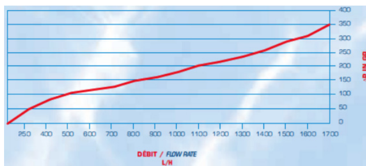
Graphe perte de charge / débit
